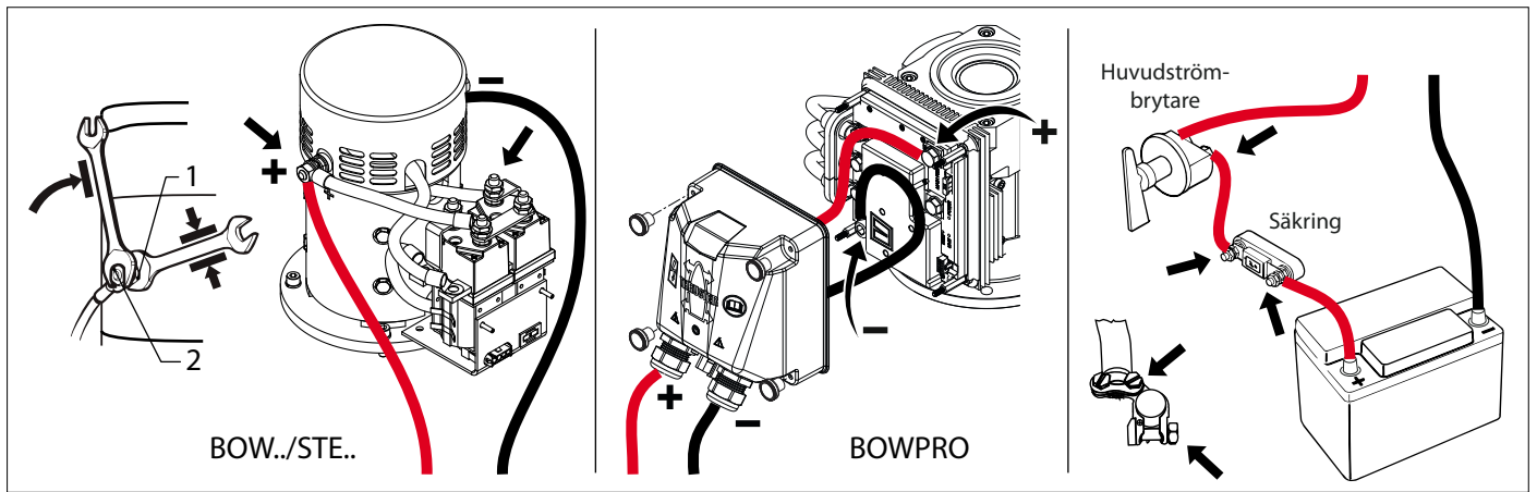
BOW-seriens /STE-seriens propellereenheter
