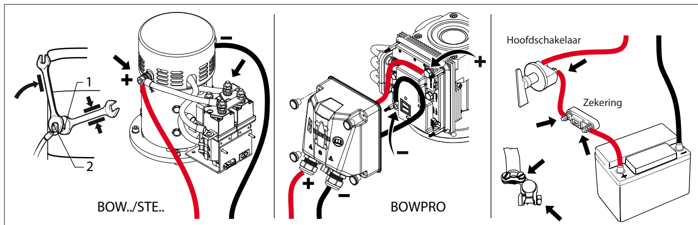
BOW / STE Serie boegschroeven
