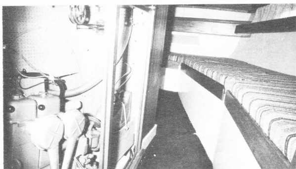
En enlevant deux panneaux dans la coursive arrière, on accède aisément au moteur
