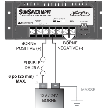
Figure 5. Câblage de la batterie.
