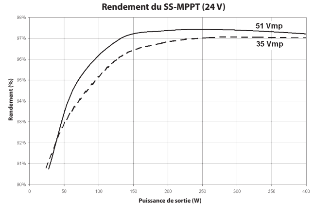
Figure 11. Courbes de rendement du SS-MPPT 24 V
