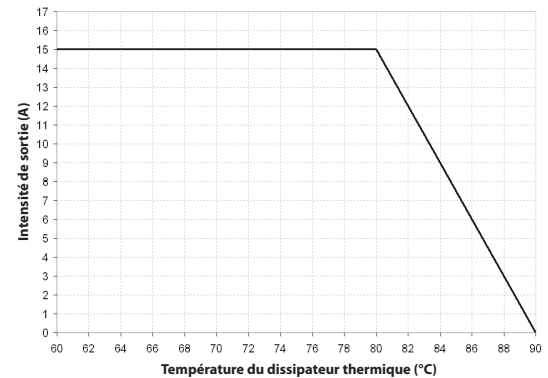
Figure 12. Intensité de sortie vs la température du dissipateur thermique
