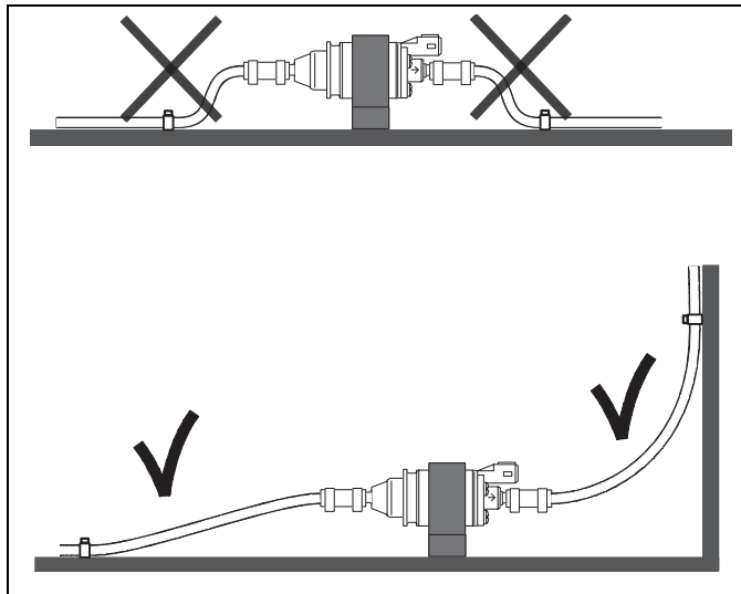
Fig. 20: Fixation de la conduite de carburant
