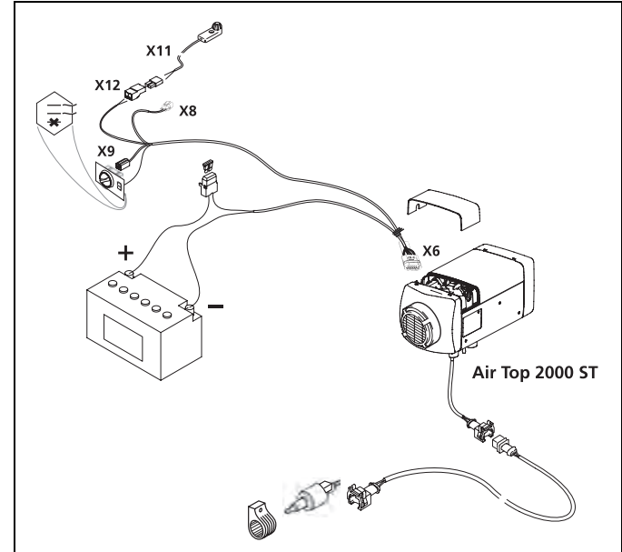
Fig. 31: Faisceau de câbles Air Top 2000 ST
