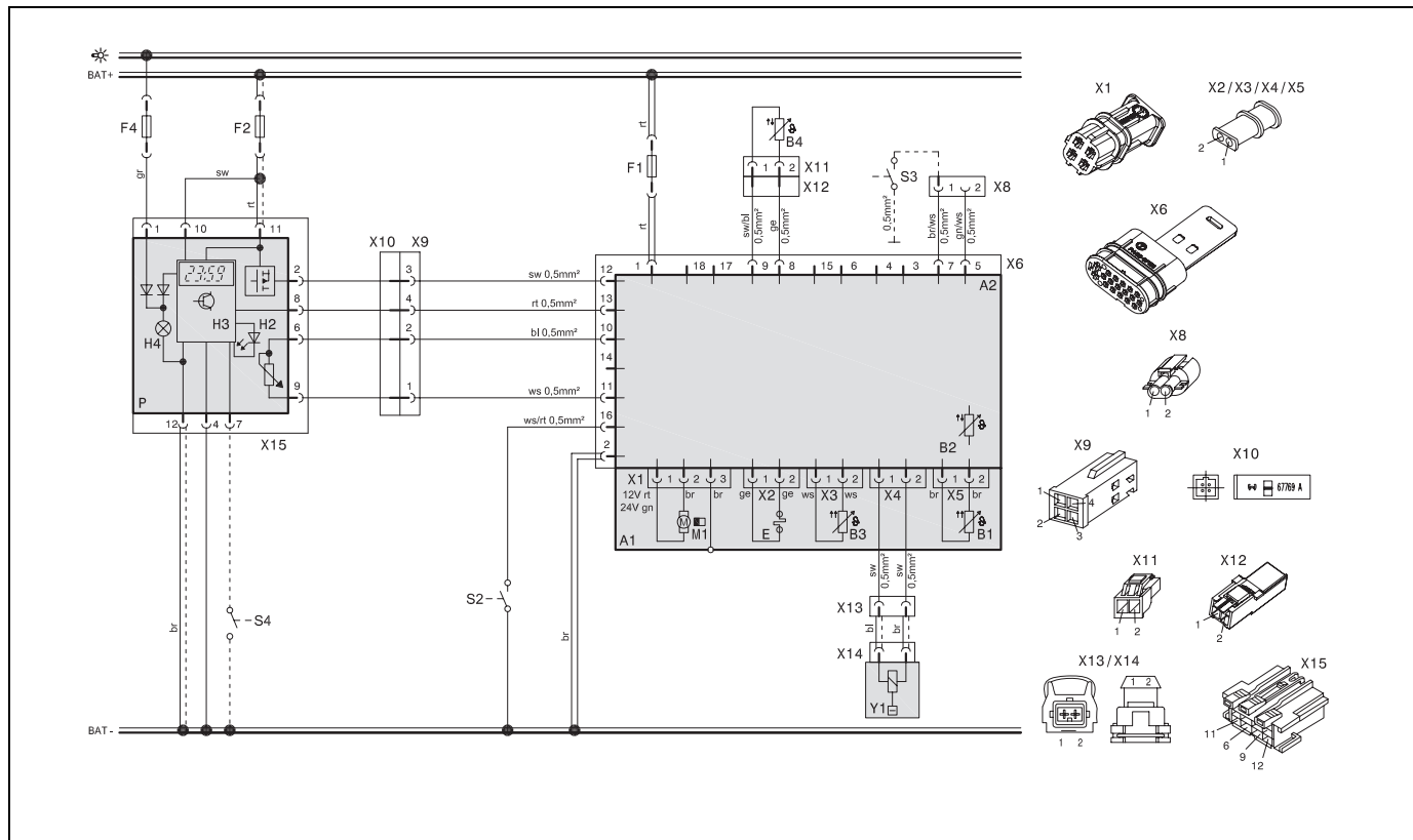
Fig. 48: Diagramme des câblages Air Top 2000 ST, 12V/24V horloge polyvalente, légende : voir pages 47 et 48
