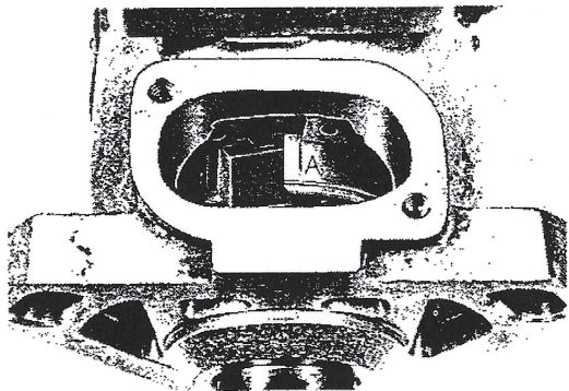
Trait repère de rotor en ligne sur l'arête de circlip
