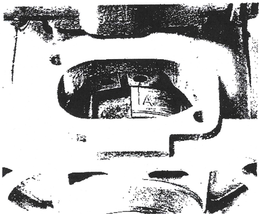
Repère sur rotor de pompe et circlip de calage (moteurs ancien modèle)
